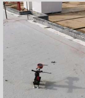
Trækprøvning ifbm. elementmontage
